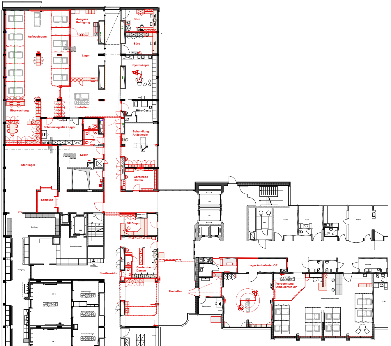
Grundriss Behandlungstrakt
